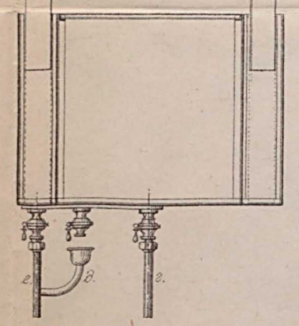
Черт. 8. Водосной разрѣзъ бака.
