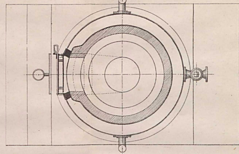
Черт. 7. Поперечный разрѣзъ подворматама.
